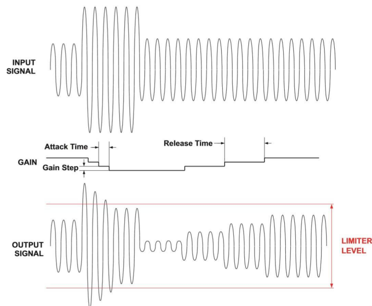
Fig. 1 Limiter Function
