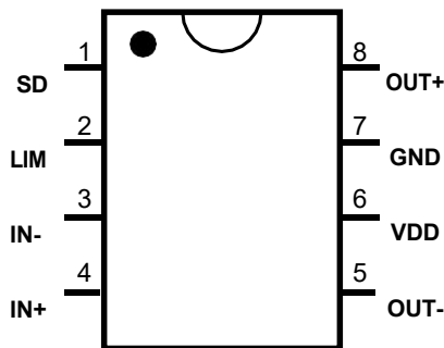
FH8863 顶视图
